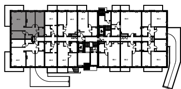
↑ RZUT KONDYGNACJI
