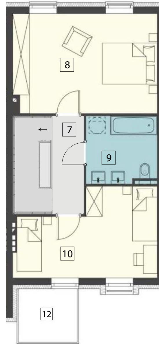
POZIOM 1
